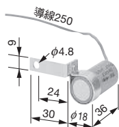
大約重量：22 g DCR2-50A22E
