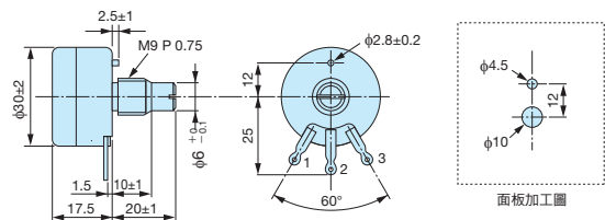
外觀尺寸 mm
