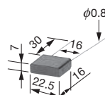
大約重量：5 g DCR2-10A25C
