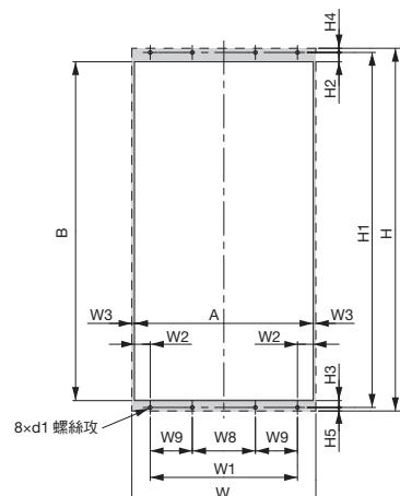
面板加工圖 8
