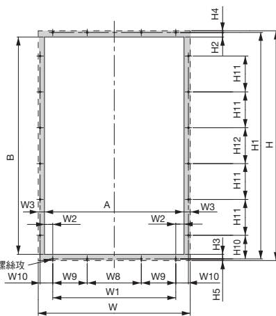
面板加工圖 7
