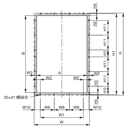
面板加工圖 6
