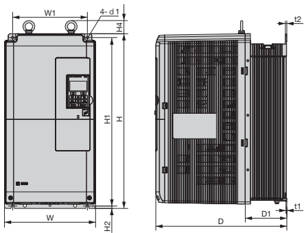
外形尺寸圖 1
